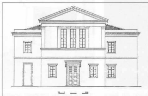
11. Η πρόσοψη του Κακουργοδικείου με τις δύο πτέρυγες, τη νότια και τη βόρεια. Σχέδιο Εμμ. Μπίρη.
