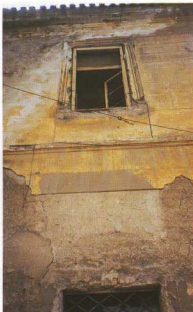
14. Παράθυρο του ορόφου στη βόρεια πτέρυγα με πλαίσιο από κοινόμα διαμορφωμένο στο επάνω μέρος σε δόντι. Σημερινή κατάσταση.
