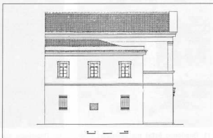
12. Η όψη της βόρειας πτέρυγας επί της οδού Κακουργοδικίου. Σχέδιο Εμμ. Μπίρη.
