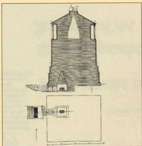
Σχέδιο του Μουσουλίου. Ο τάφος του βασιλιά βρισκόταν χαμηλό, μέσα στη βάση του οικοδομηματος, για να είναι καλύτερα προστατευμένος. Την είσοδο σφράγιζε μια μεγάλη πέτρα. Το ύψος του Μουσουλίου έφτανε τα 42 μέτρα, ήταν δηλαδή ψηλότερο από τον Πάρθενωνα. Η βάση του ήταν κατασκευασμένη από 8 πατώματα!
